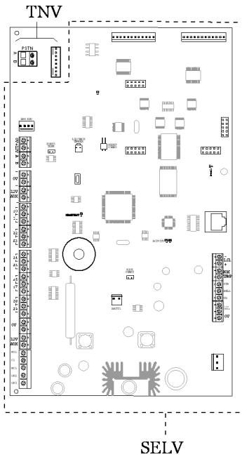
TNV – Connecteur ligne téléphonique. SELV – Autres connecteurs.
