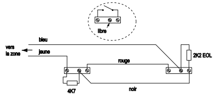
Figure 28 Exemple : Double contact sur la même zone supervisée.
