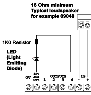
Figure 31 Sorties de l'extension.
