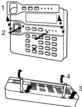
Figure 6 Ouverture du clavier
