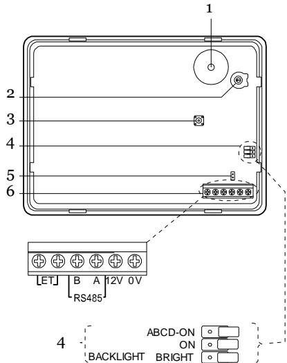
Figure 7 Face arrière du clavier
