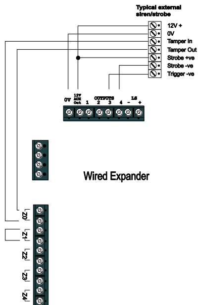
Figure 32 Câblage sirène AP NF sur extension
