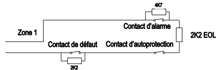
Figure 29 Exemple : Câblage d'une Zone masquage, méthode à trois résistances.
