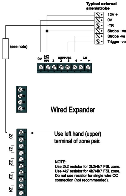
Figure 33 Câblage sirène AP ZFS sur extension.
