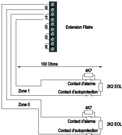
Figure 26 Câblage des zones avec résistances sur l'extension
