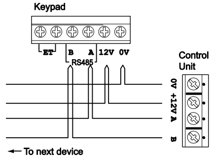
Figure 20 Connexion du clavier
