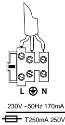
Figure 22 Connexion secteur
