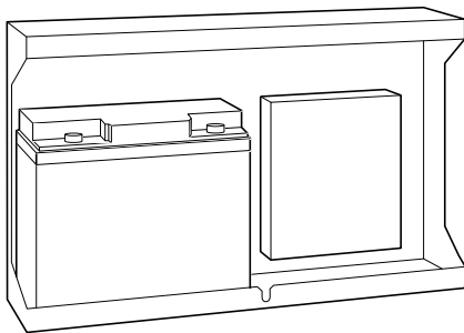
Figure 37 Mise en place de la batterie
