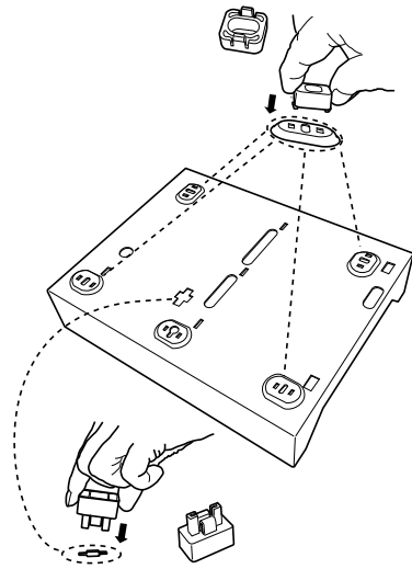
Figure 13 Cales de fixation et glissière d'AP.
