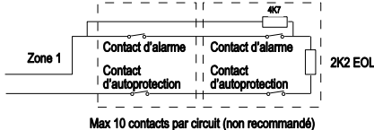
Figure 27 Câblage de deux détecteurs sur une zone supervisée.
