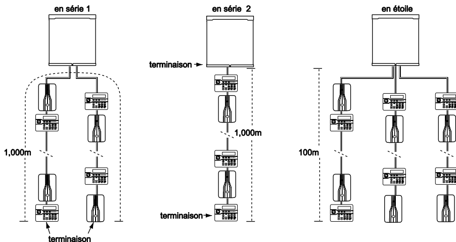
Figure 11 Type de Configurations de câblage du bus
