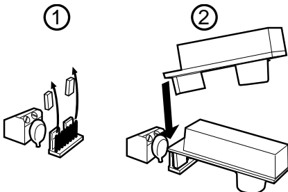
Figure 35 Mise en place du filtre ADSL01.
