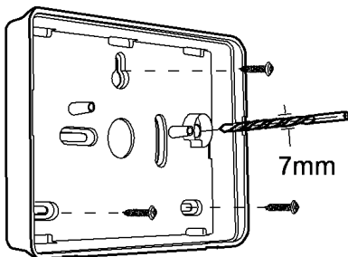
Figure 19 Fixation du socle clavier
