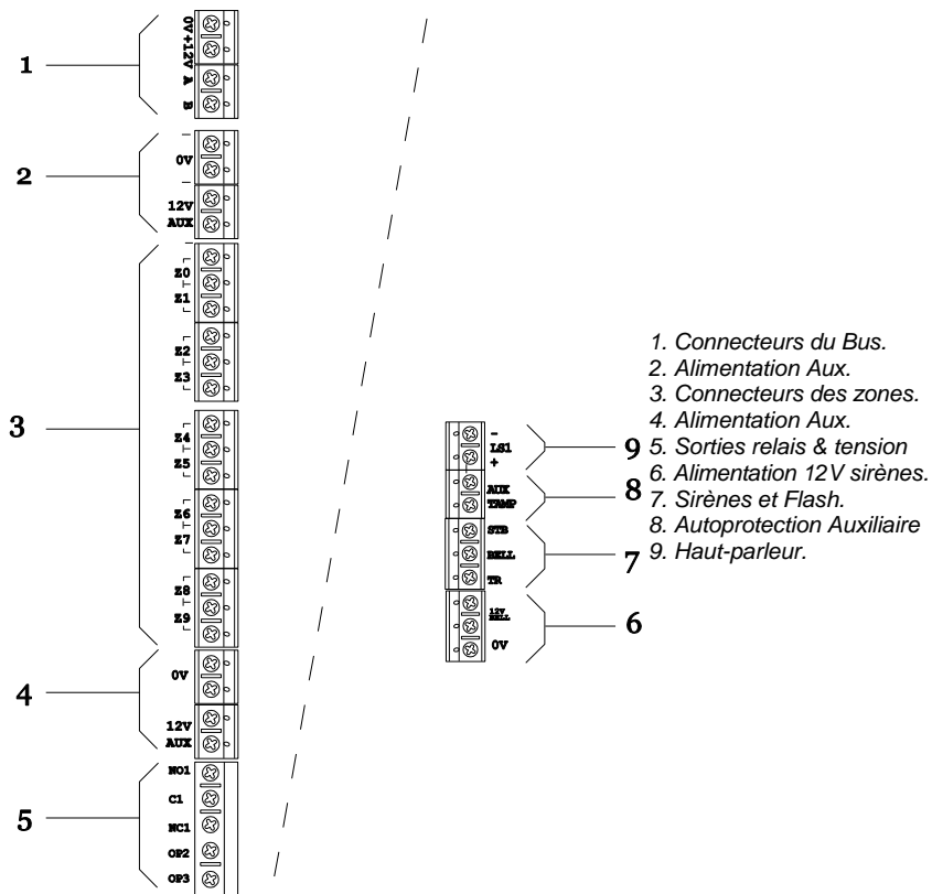
Figure 4 Connecteurs de la centrale
