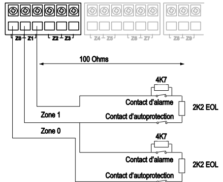
Figure 25 Câblage des zones avec résistance sur la centrale
