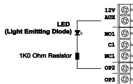
Figure 30 Connexion Sirène & Voyant
