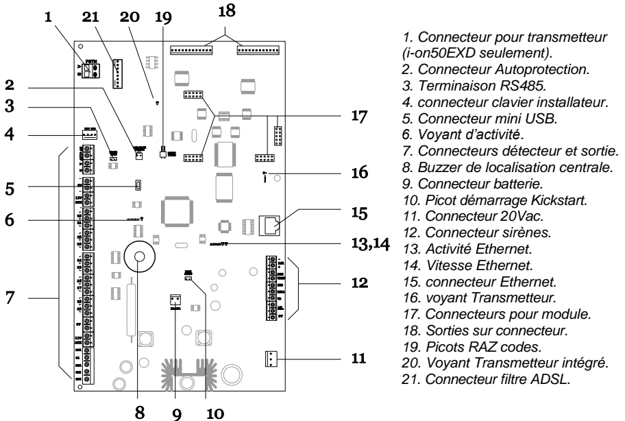
Figure 3 Circuit électronique de la centrale
